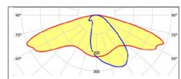
mod. LIOX
