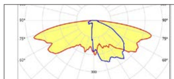
mod. LIOX
